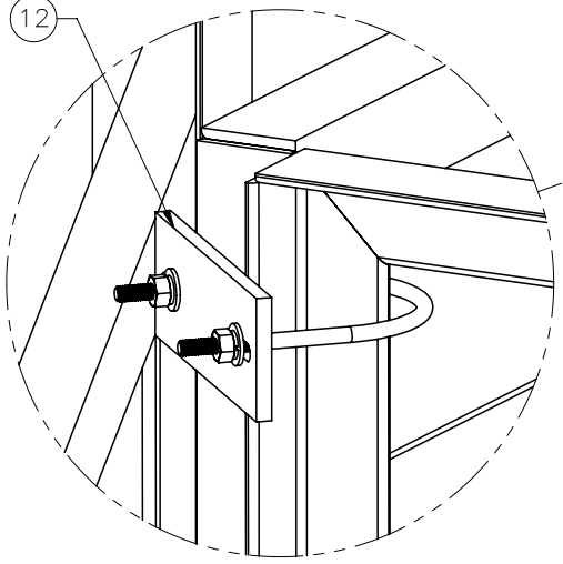
CORNER BRACKET DETAIL TYP 3X
