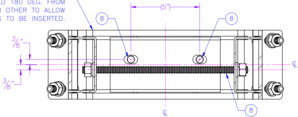
SECTION A-A 1
